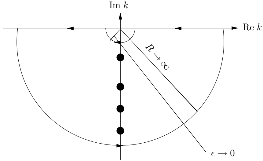
Abbildung 3: Zum Levinsontheorem
