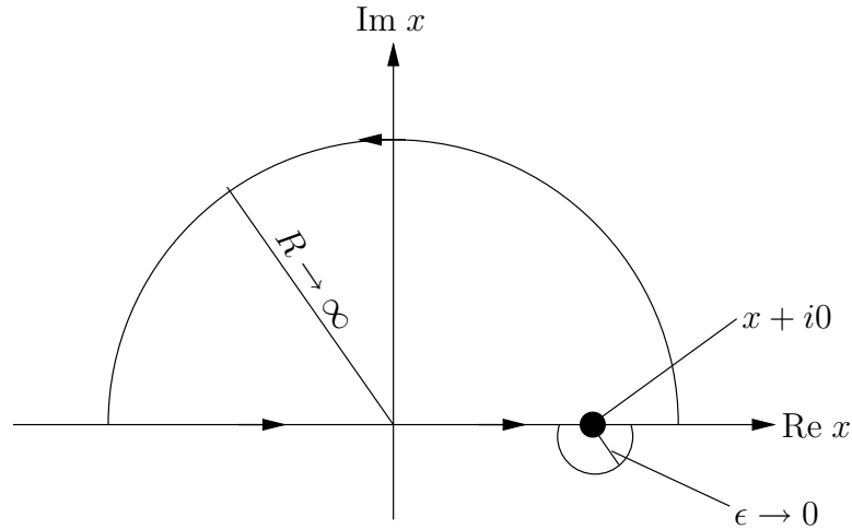
Abbildung 1: Zum Beweis von (63)
