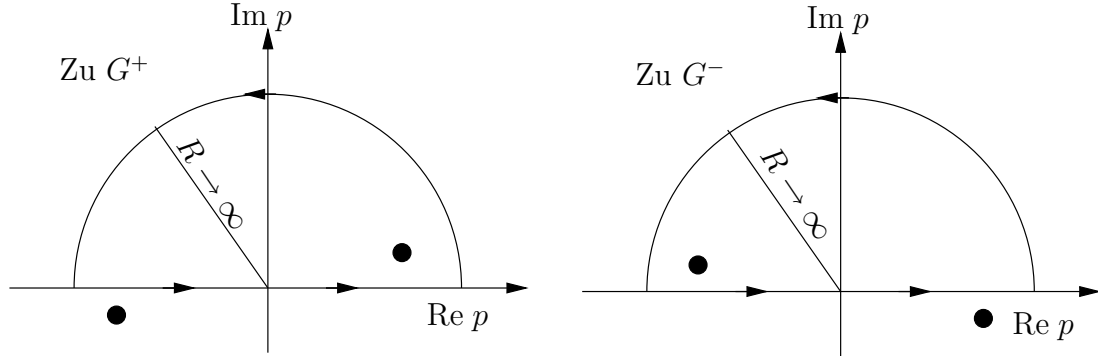
Abbildung 2: Zur Berechnung der freien Greenfunktionen
